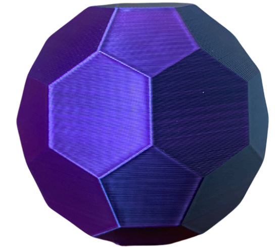
ICOSAEDRO TRUNCADO
