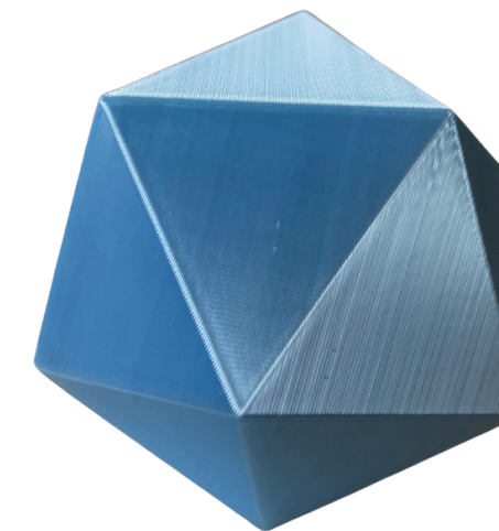
ICOSAEDRO
