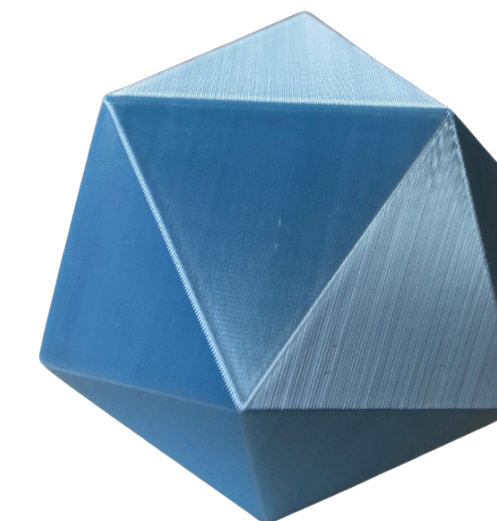
ICOSAEDRO
