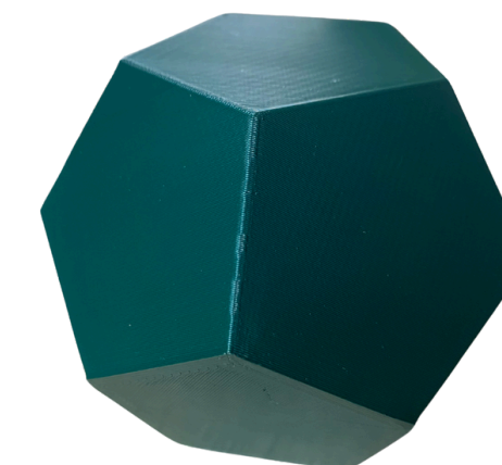
DODECAEDRO
