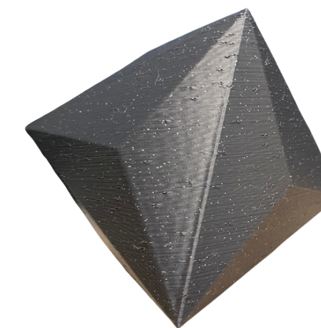
TRIAKISICOSAEDRO
